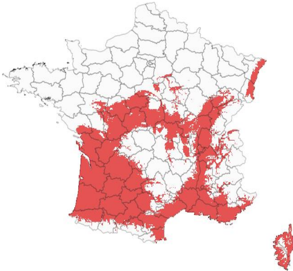
Figure 8 : Prédiction des zones au climat potentiellement favorable pour un établissement de Xylotrechus chinensis basées sur des approches d'enveloppe climatique en France (en rouge sur la carte).
