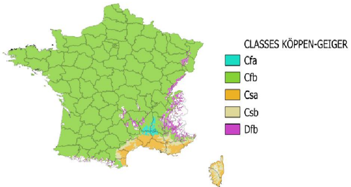
Figure 6: Zones climatiques Köppen-Geiger considérées comme potentiellement favorables pour l'établissement de Xylotrechus chinensis en France. Les régions géographiques colorées en blanc ne sont pas considérées comme potentiellement favorables.
